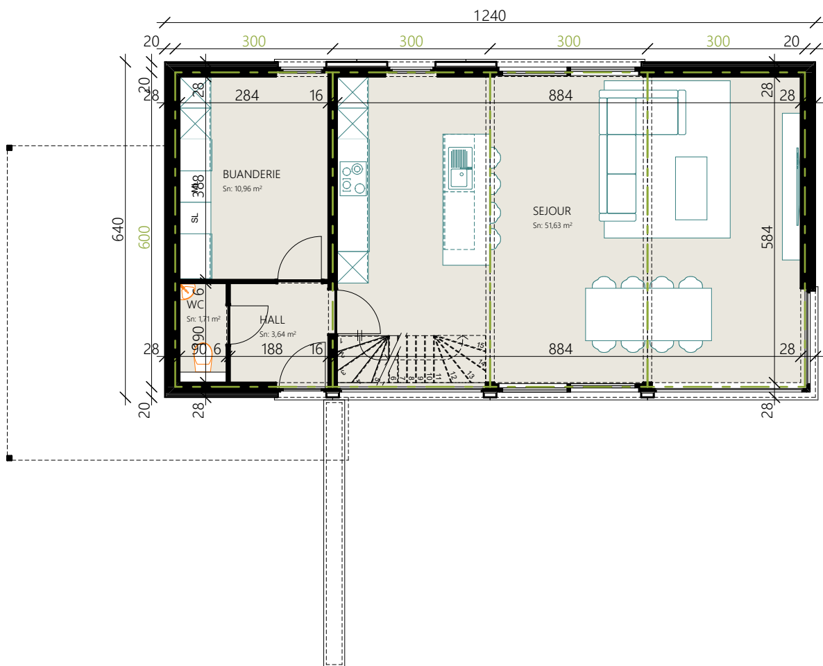
REZ-DE-CHAUSSEE
