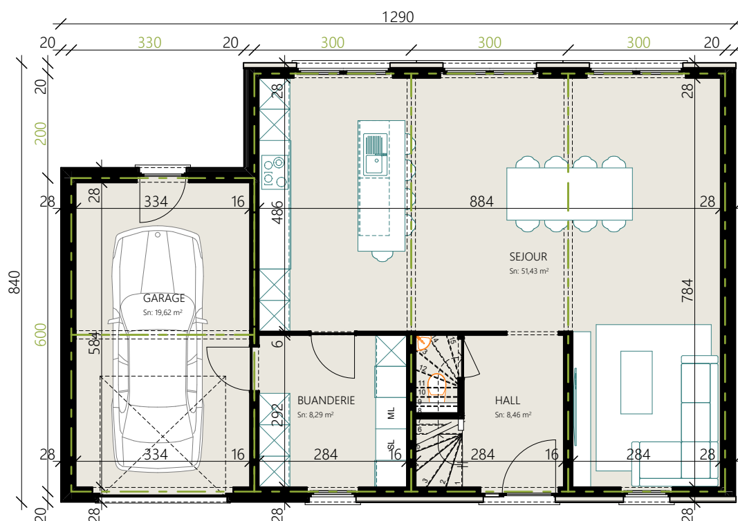
REZ-DE-CHAUSSEE
