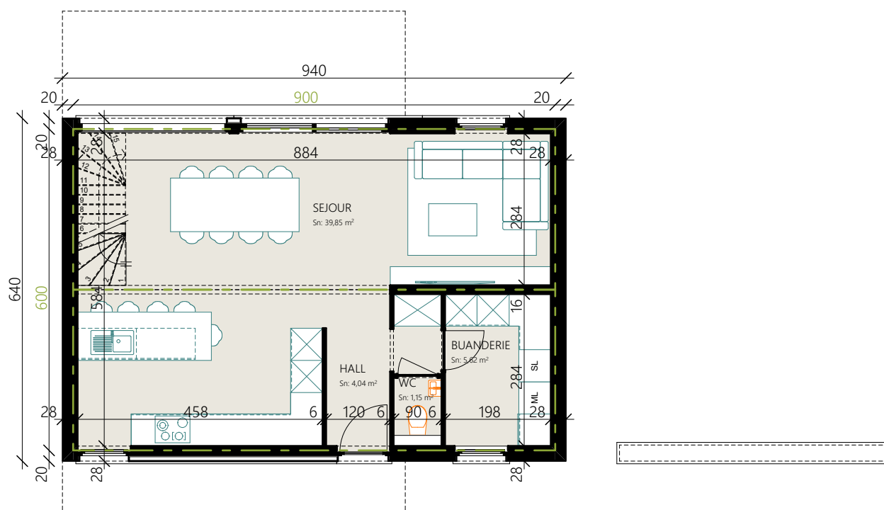
REZ-DE-CHAUSSEE
